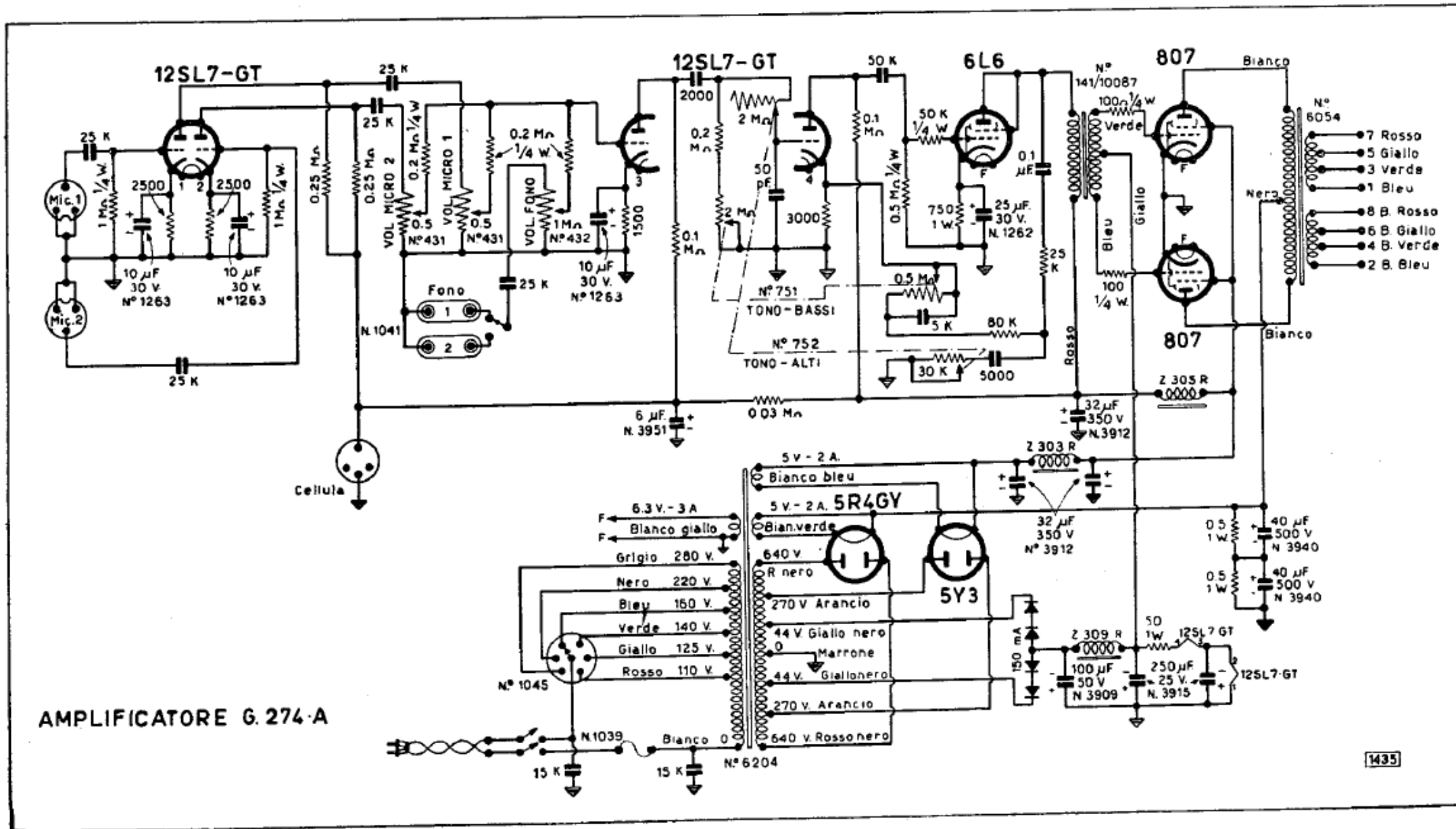
Lo schema elettrico.
